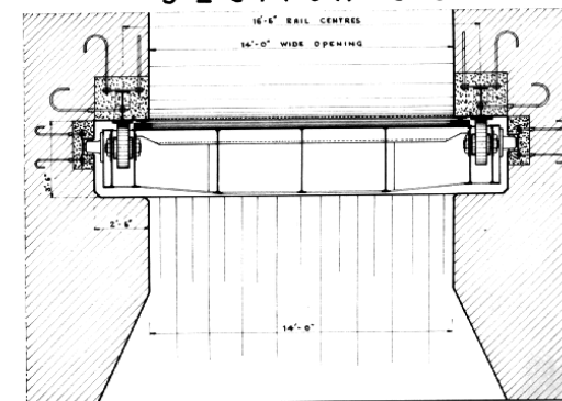
SECTION D-D
