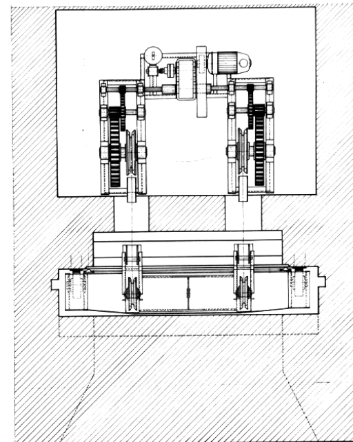
SECTION D-D
